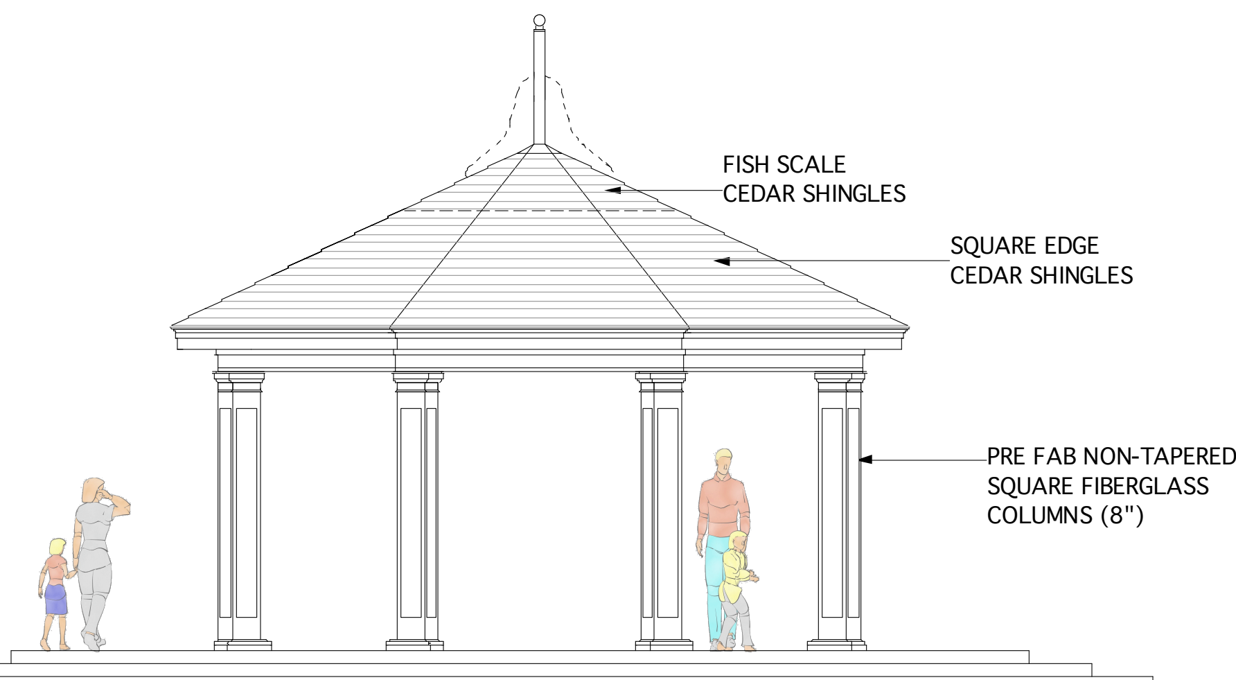
ELEVATION
